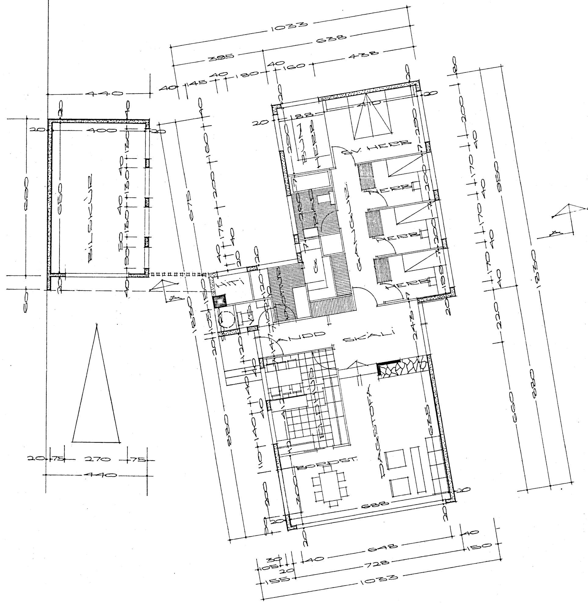
GRUNNMYND HÚSS.
