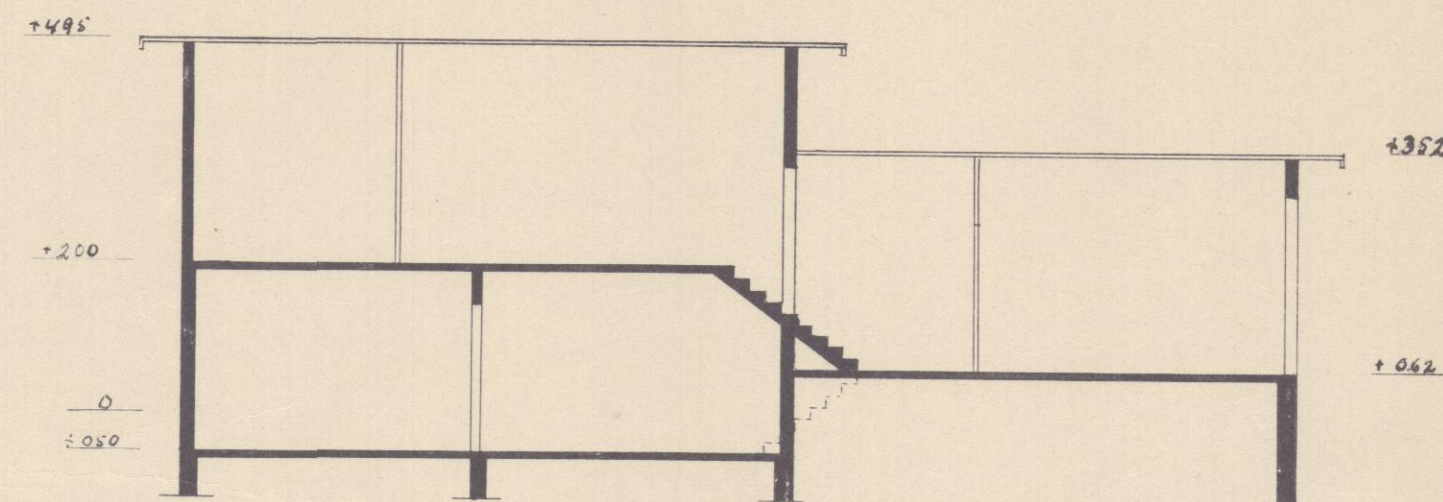
Skurður
