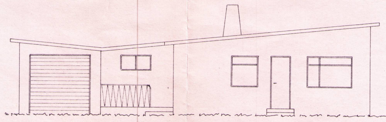
NORÐURHLIÐ
