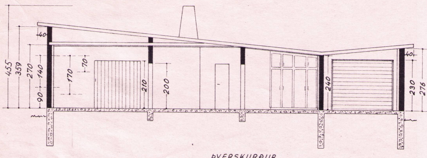
ÞVERSURÐUR
