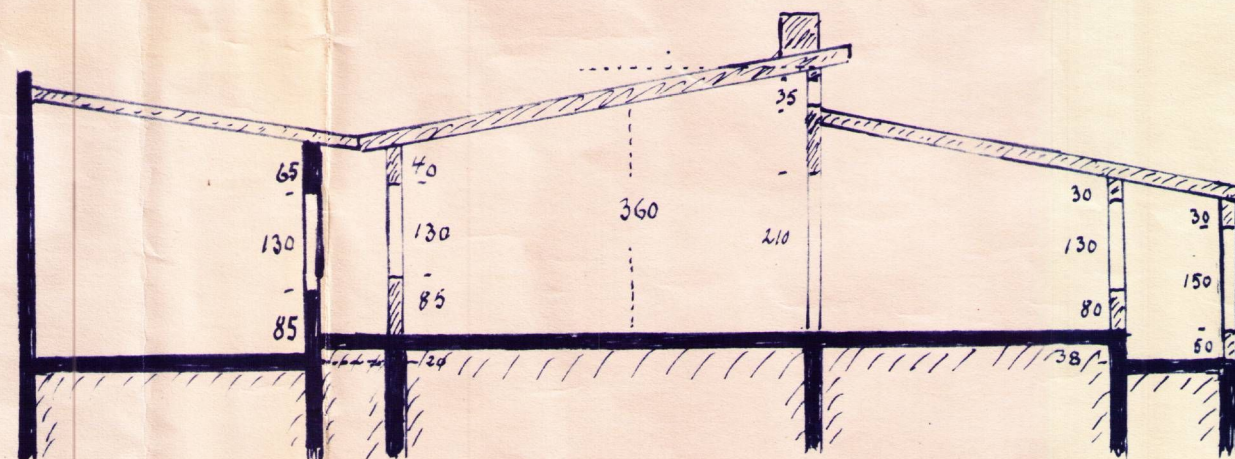
ÞVERSKURÐUR
