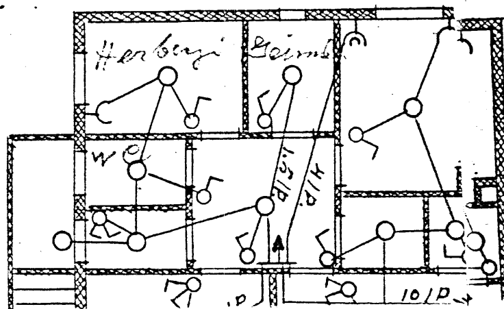
KJALLARI HITALÖGN.
