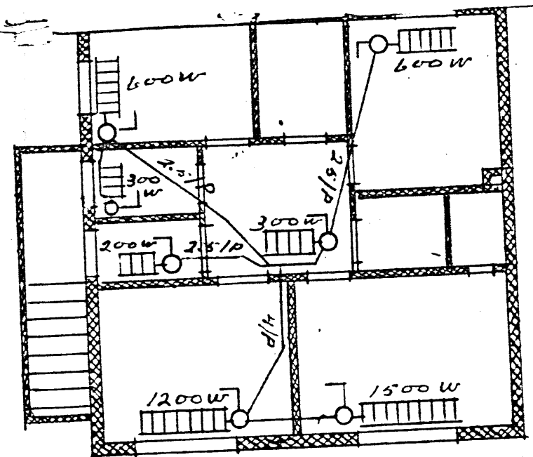
1. HÆÐ HITALÖGN
