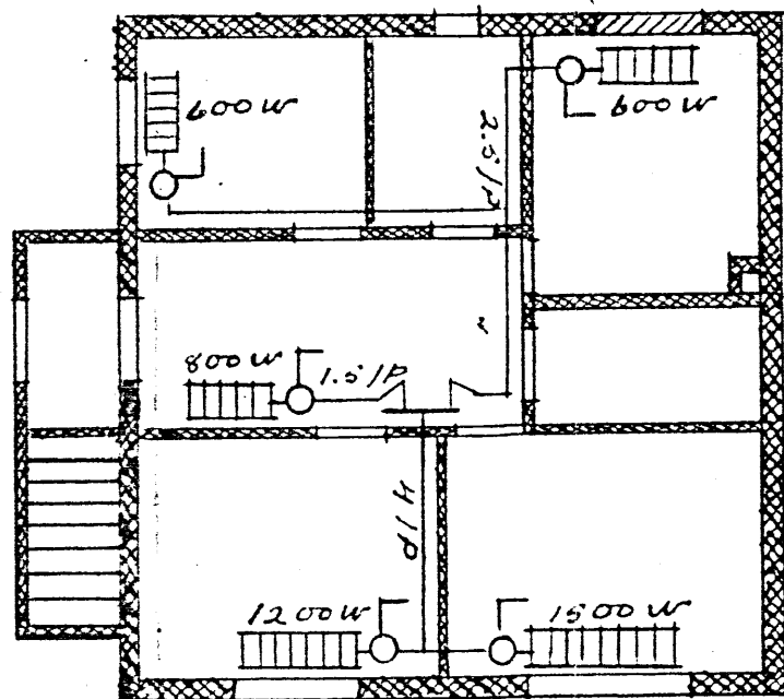
KJALLARI HITALÖGN.
