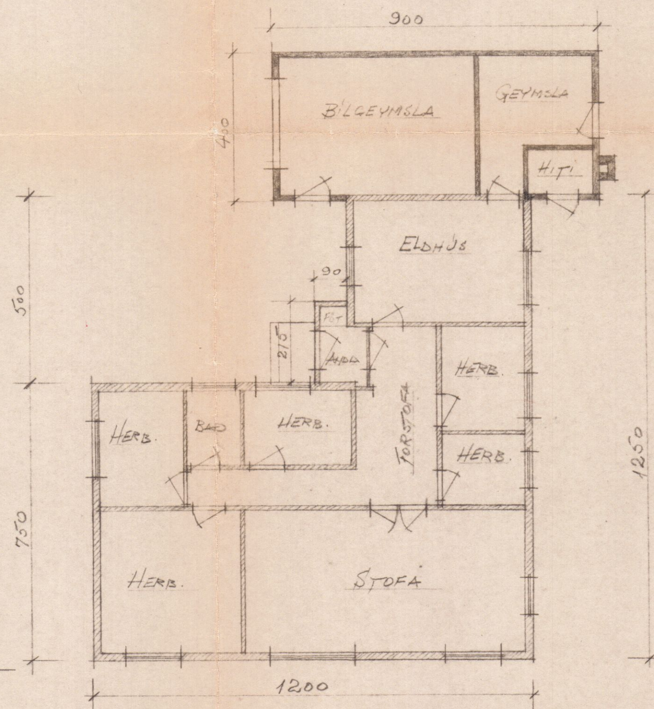
GRUNNMYND
