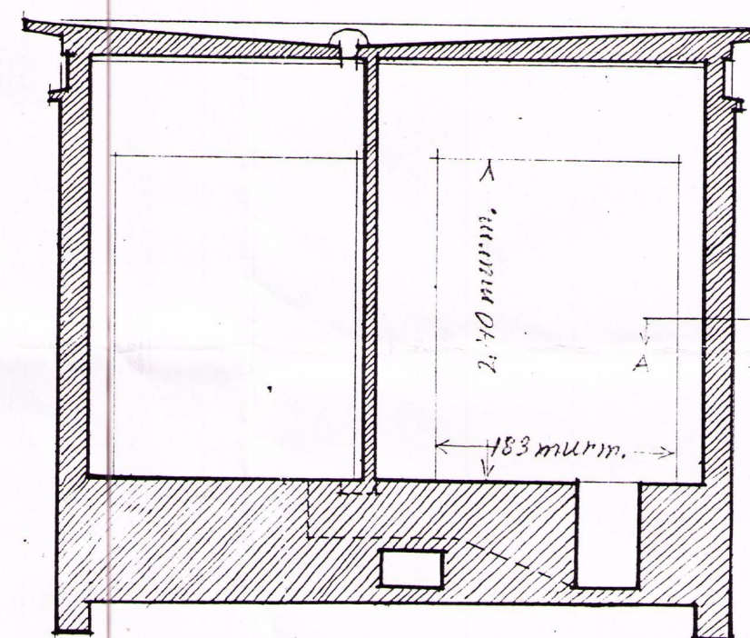
SNEIDING A-B
