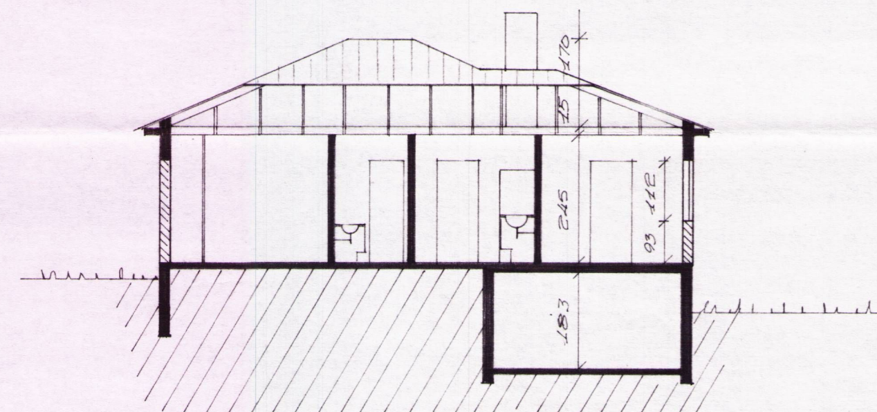
SNEIÐING A-A
