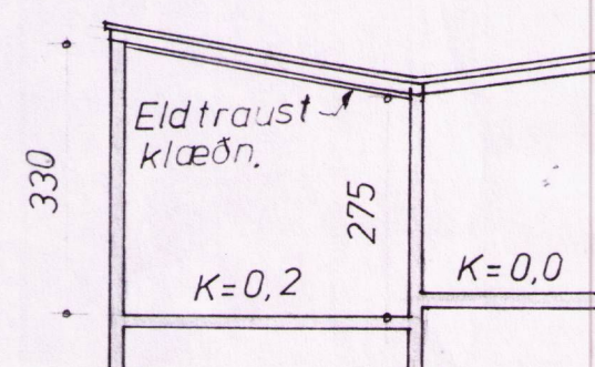
Snið m=1:100
