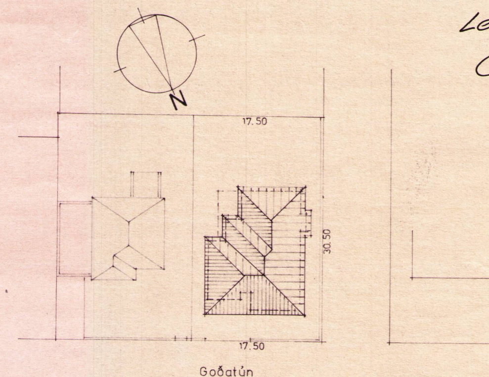
afstöðmynd 1:500
